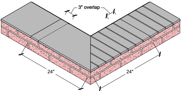
CORNER MITER
